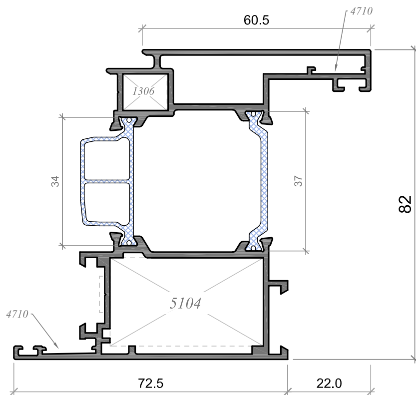
Hoja balconera alg 75
