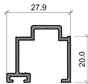
Acople Inf. Manguetón
