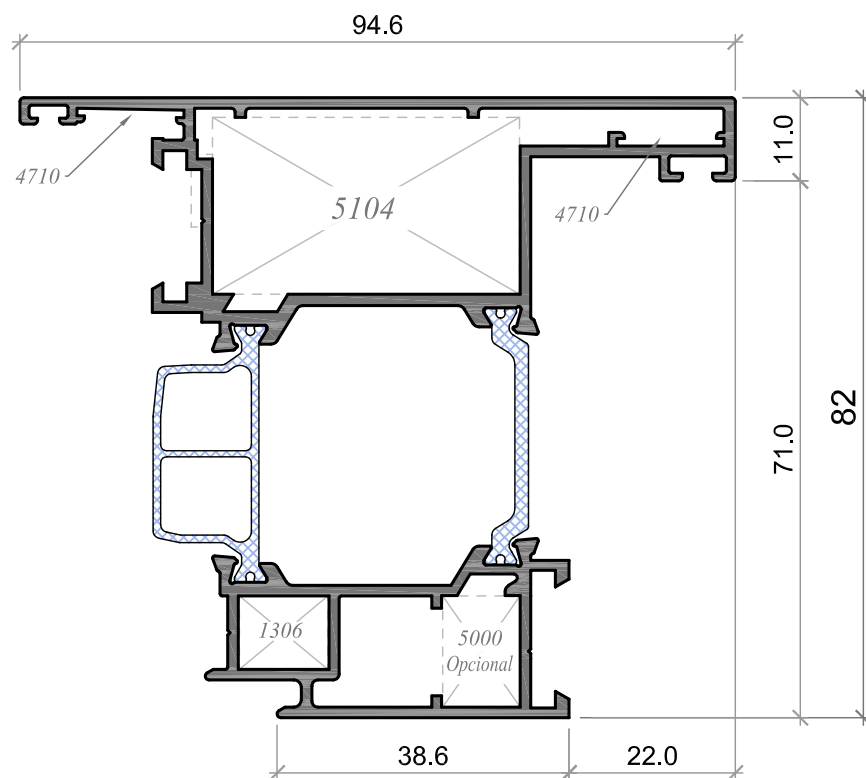
Hoja apertura externa alg 75
