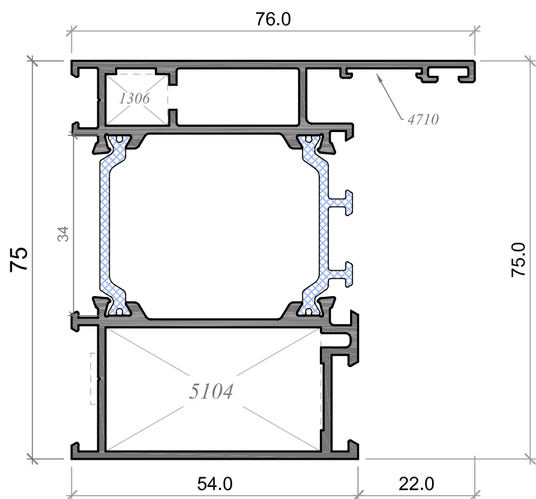
Cercos balconera alg 75
